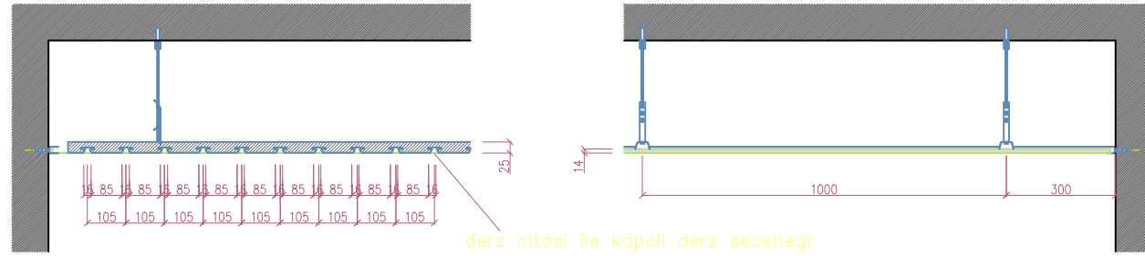
KESIT A
